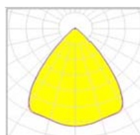
Ángulo Apertura 90°
